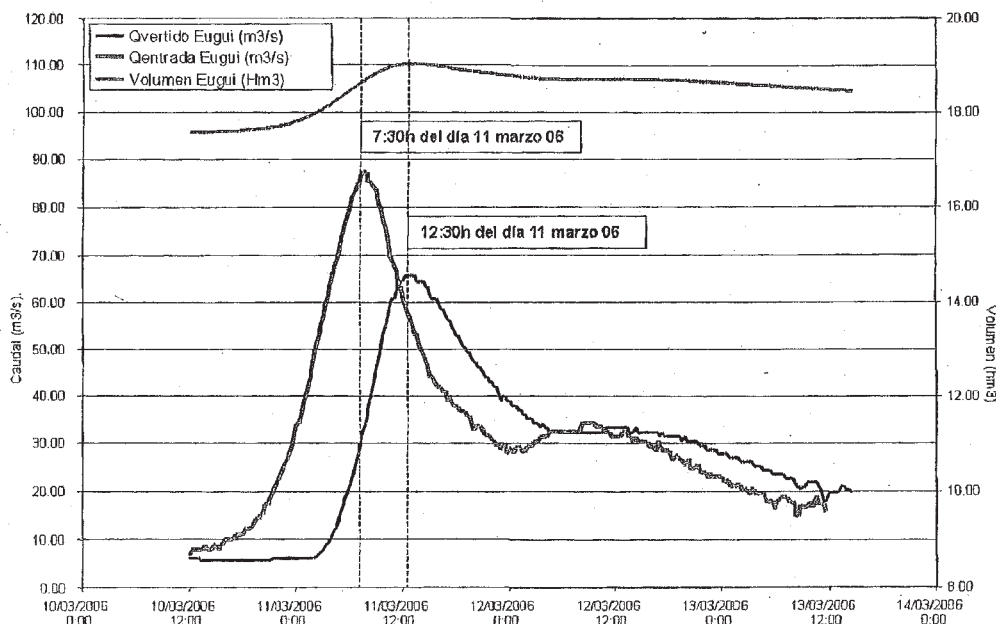
Evolución del volumen y caudales de entrada y salida en el Embalse de Eugui durante la crecida del 11 de Marzo
