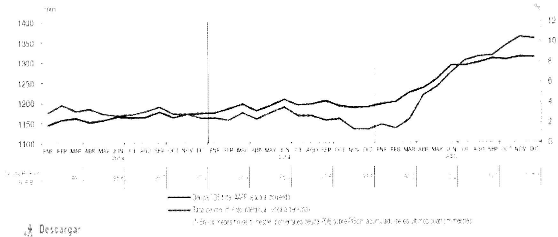
DEUDA PDE DE LAS AAPP Y TASA DE CRECIMIENTO INTERANUAL
